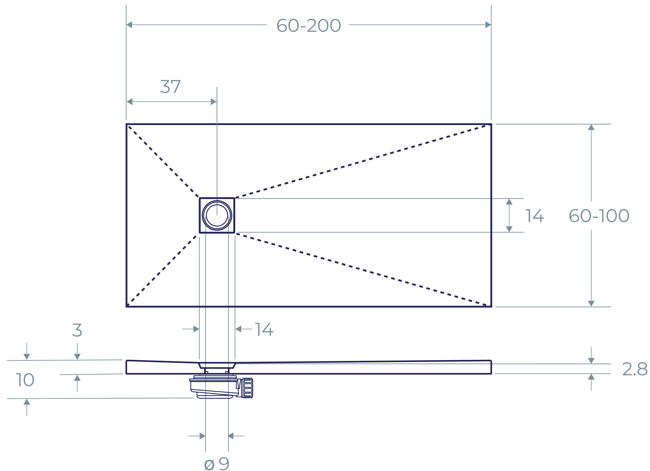
1 Floor plan and elevation / Grundriss und Aufriss / Plan et élévation / Planta y alzado / Pianta e altimetria (cm)
